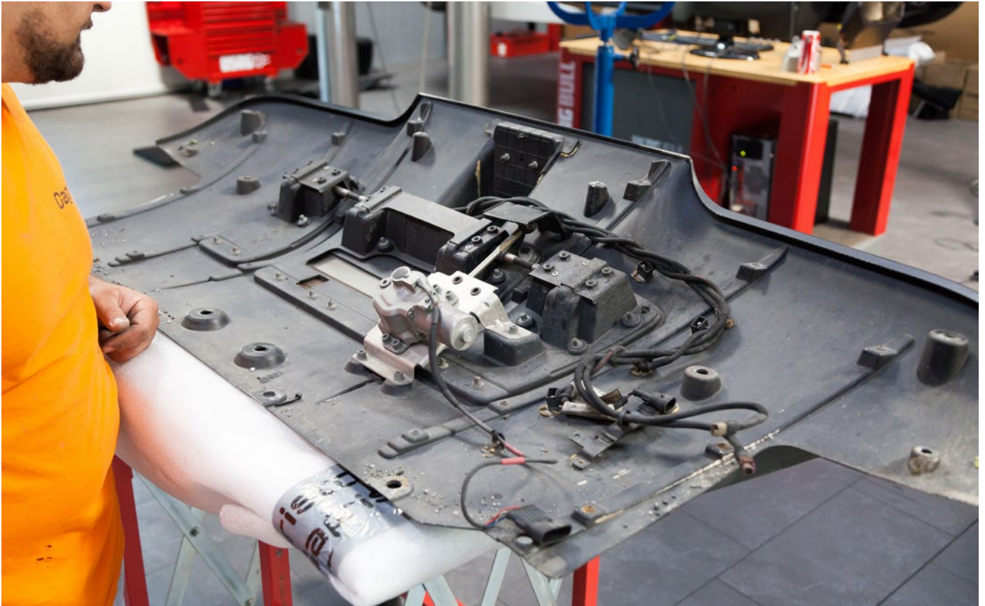
Demontierter OEM Diffusor vor der Demontage der Anbauteile. / Demounted OEM diffuser prior to the disassembly.
