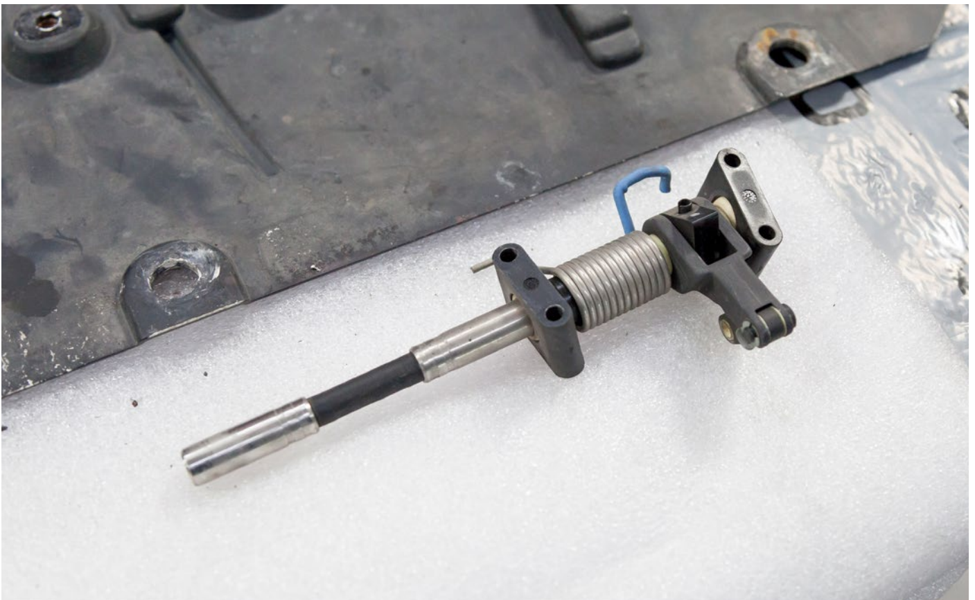
Die erste Achse ist demontiert. / The first axis is demounted.
